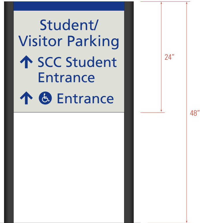
SIDE A - LOC: 10a SCALE: 1" = 1'-0"
