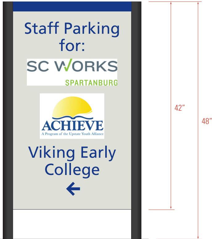
SIDE A - LOC: 2 SCALE: 1" = 1'-0"
